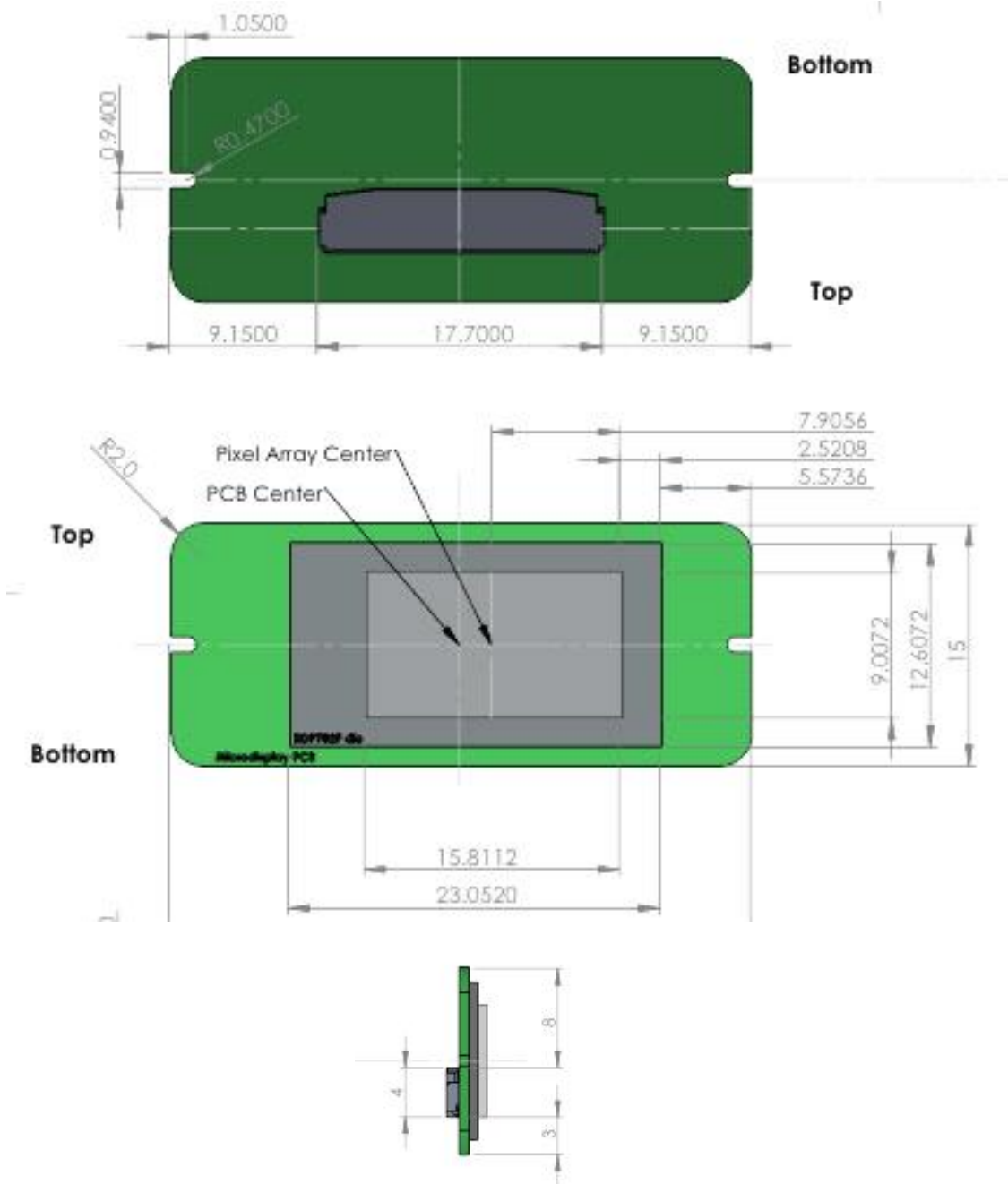
<OLEDoS Module PCB 디자인>
