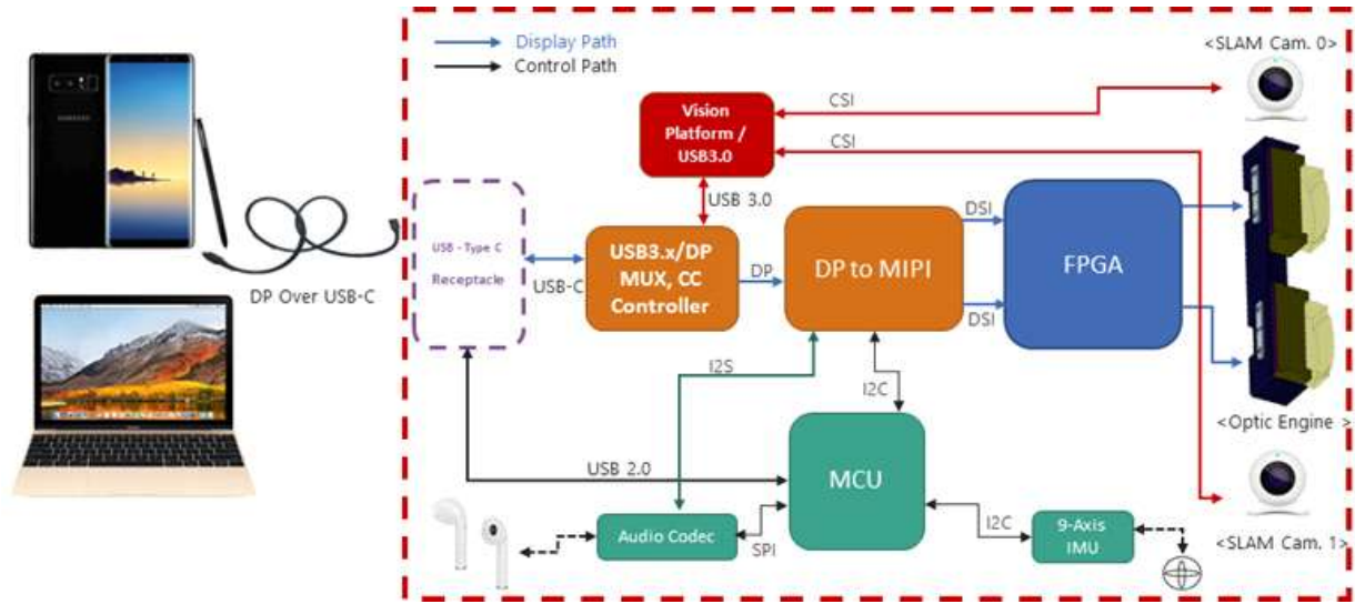
<OLEDoS EVBD 기본 개념도>
