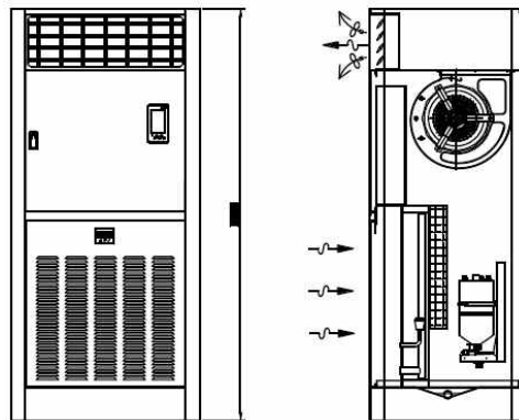
그 림 2. 향온향습기 실내기
