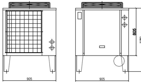
그 림 1. 향온향습기 실외기
