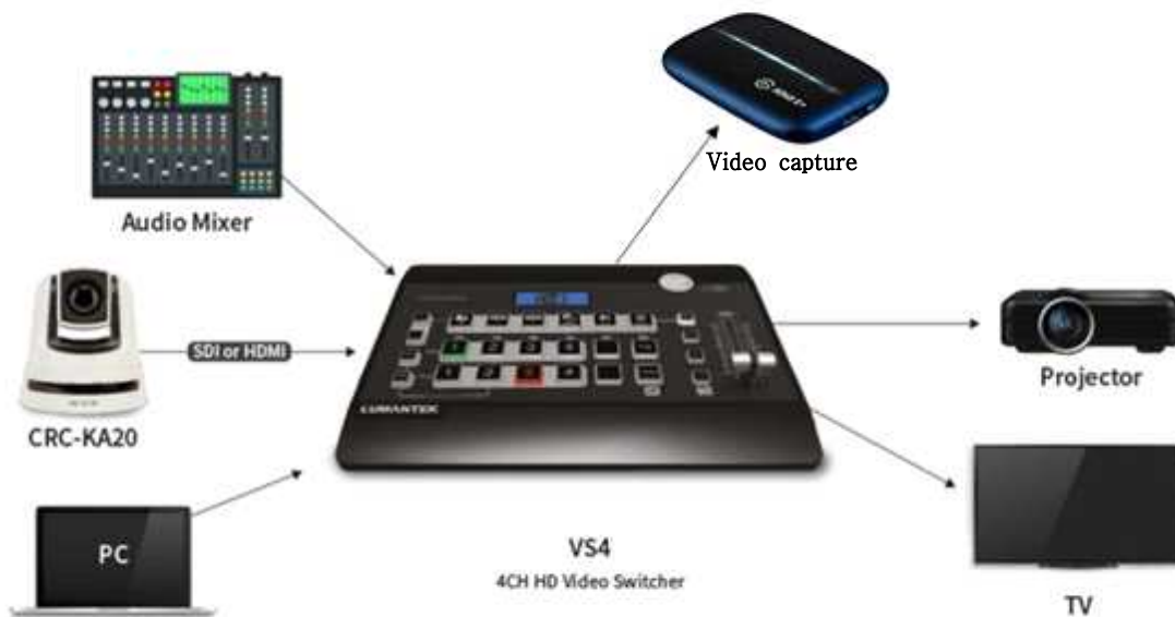
그림 1. 비대면 영상회의 시스템 구성도(PC, Projector 기보유)
