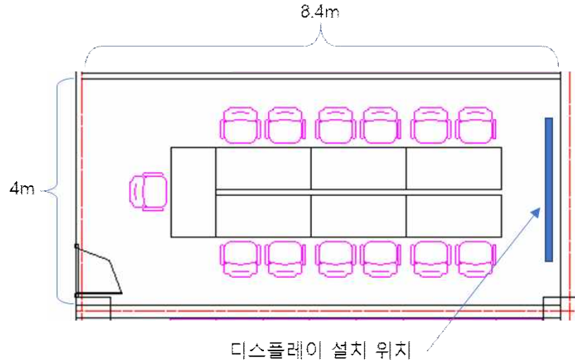
그림 2 설치공간(회의실) 도면
